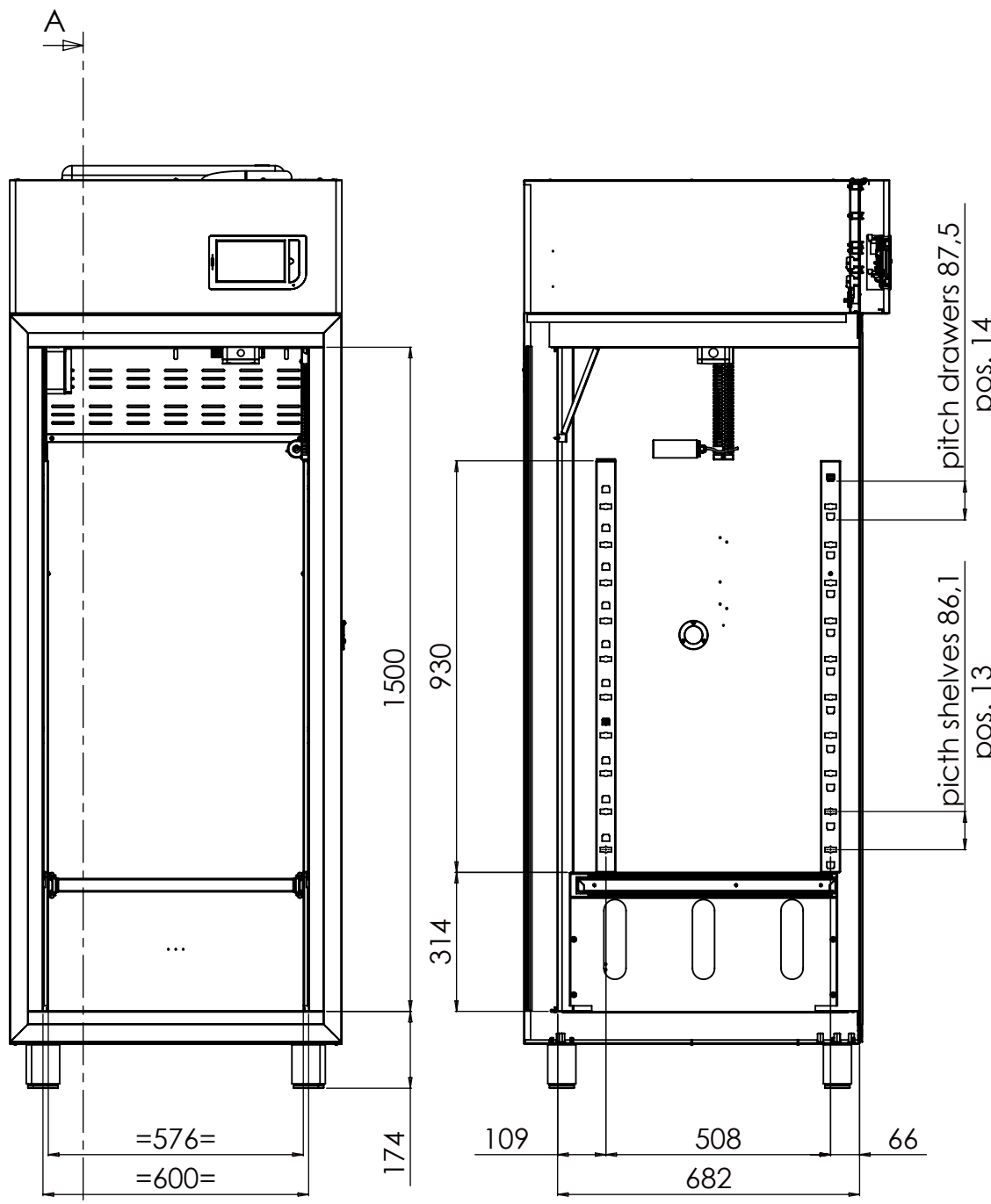
SECTION A-A
