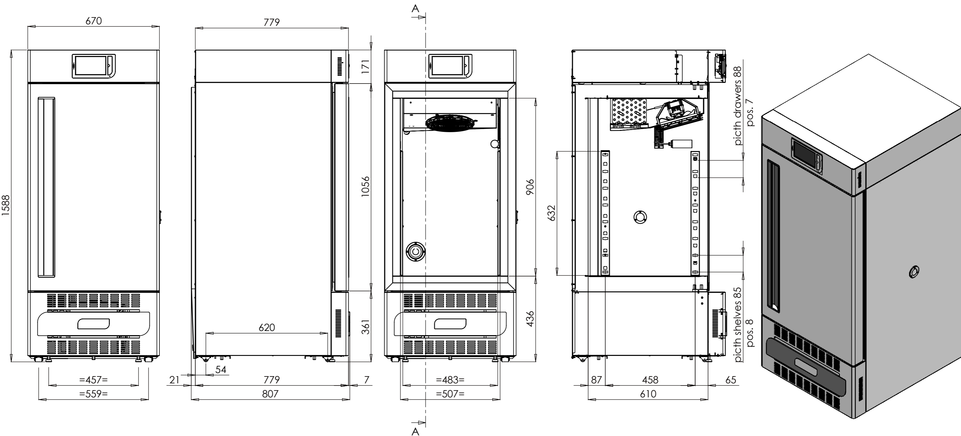
SECTION A-A
