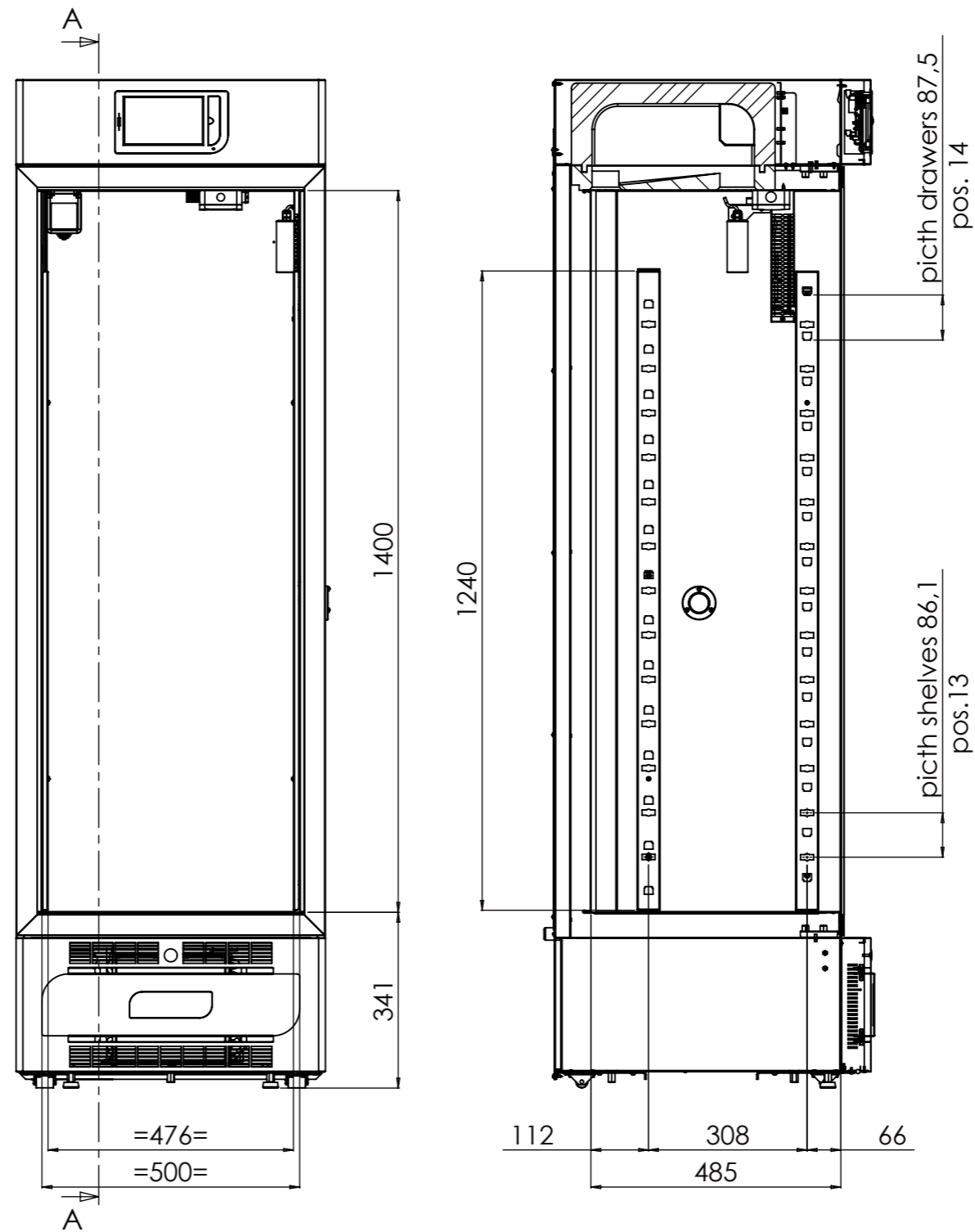
SECTION A-A
