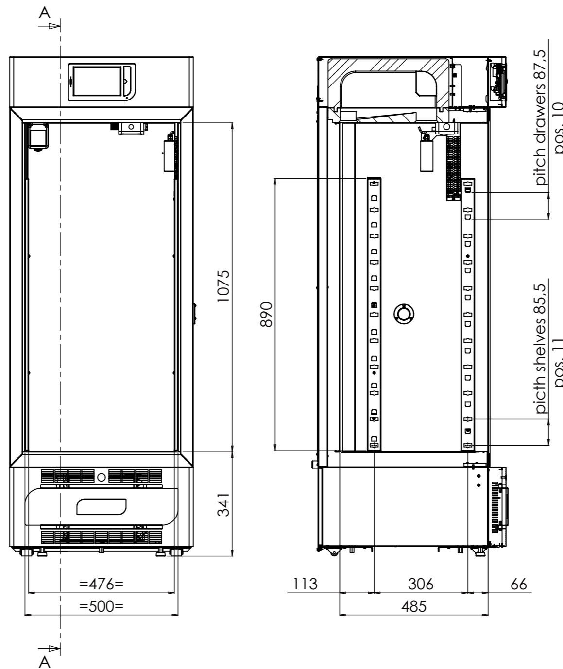
SECTION A-A
