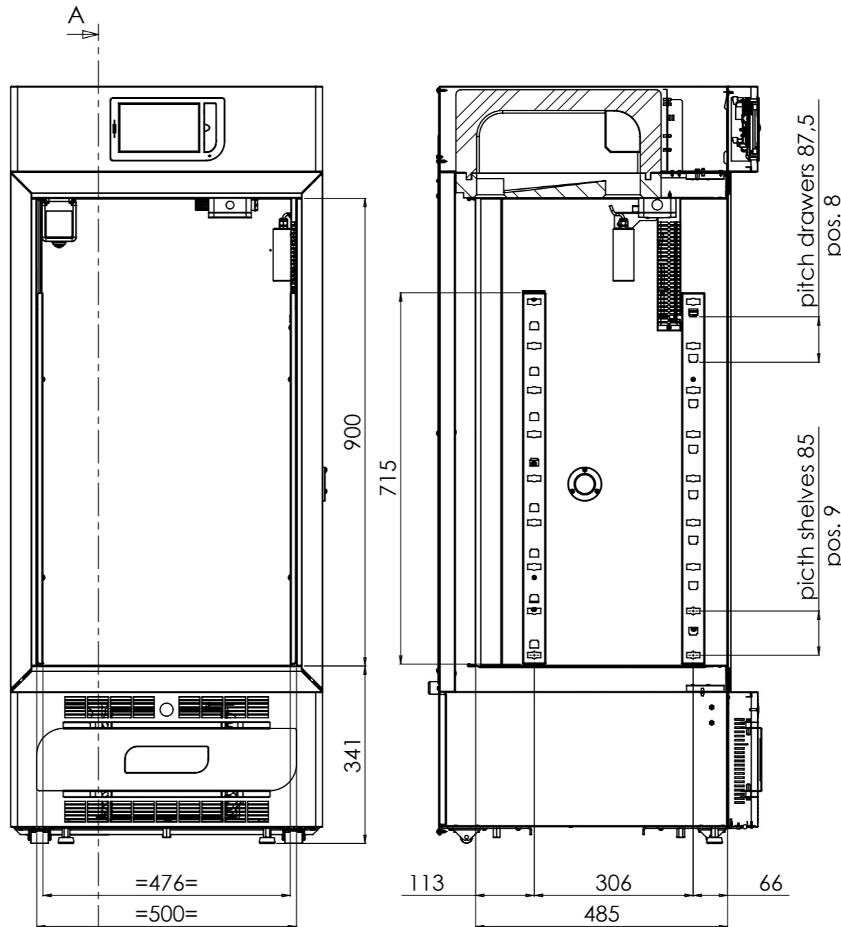
SECTION A-A
