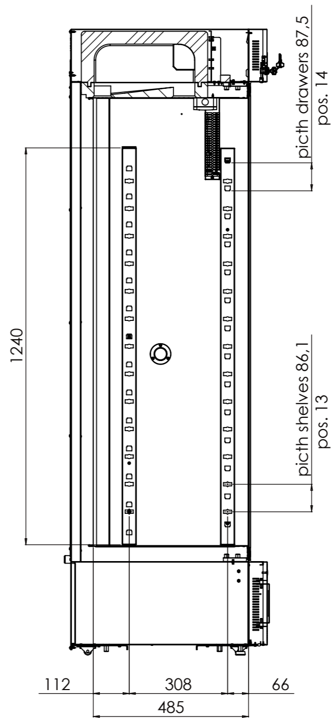
SECTION A-A
