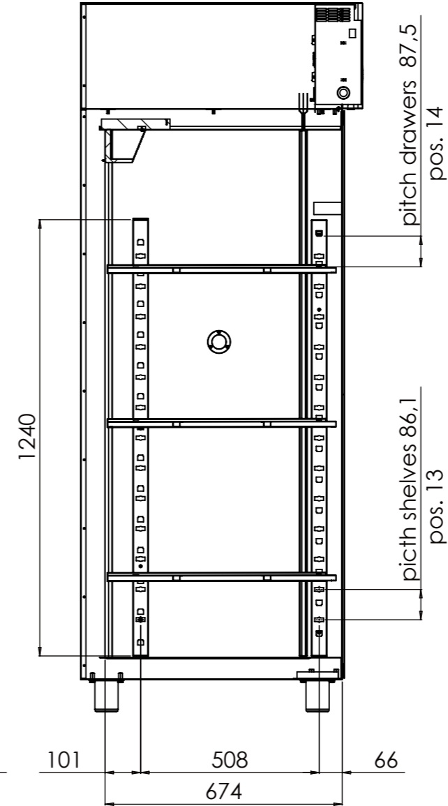
SECTION A-A
