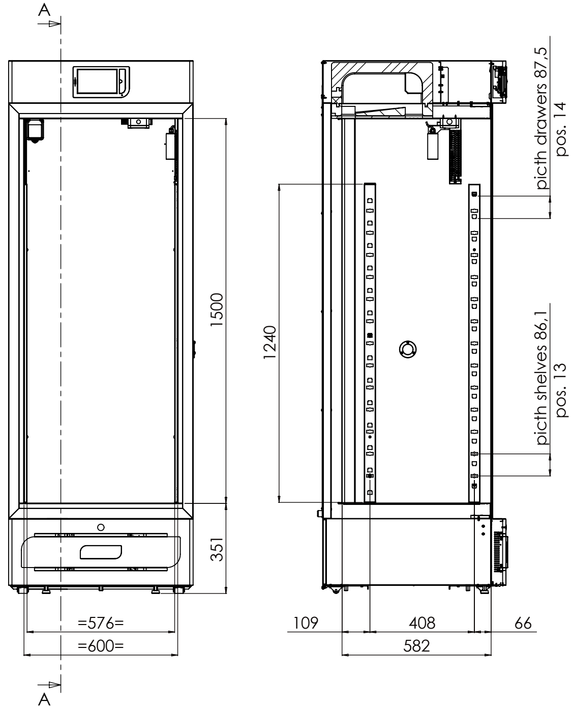
SECTION A-A
